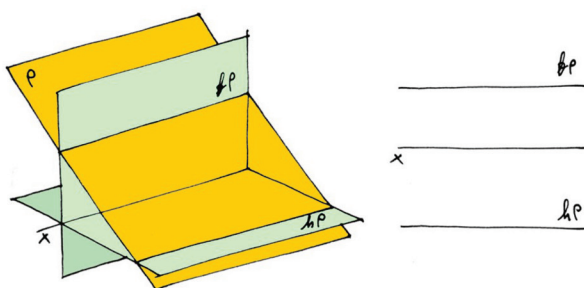
Plano de rampa
