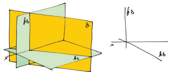
Plano vertical ou projectante horizontal
