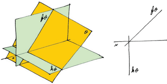
Plano de topo ou projectante frontal
