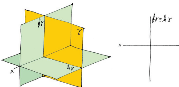
Plano de perfil
