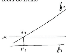
Recta frontal ou recta de frente
